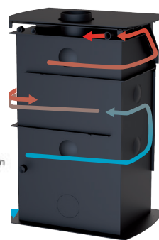
Vand-cirkulationen
